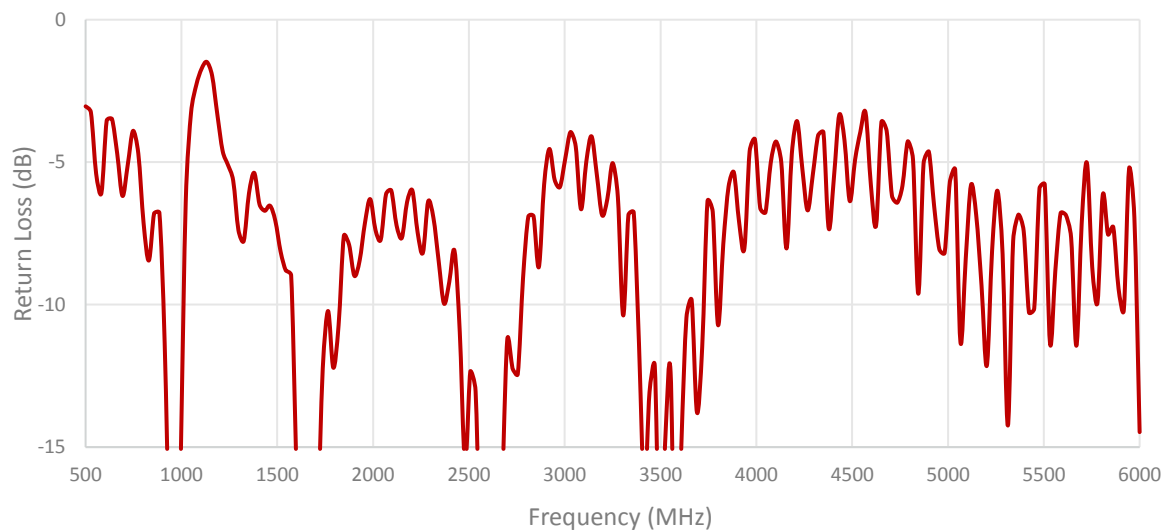
Cable 2: 5GNR
