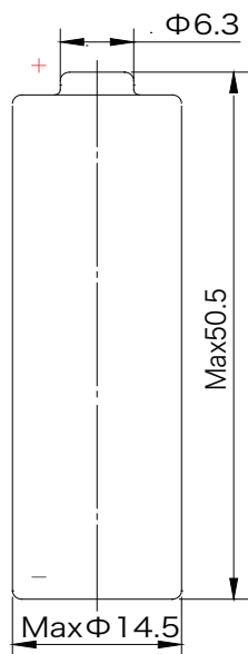
Dimensions in mm (GB1804-m)
