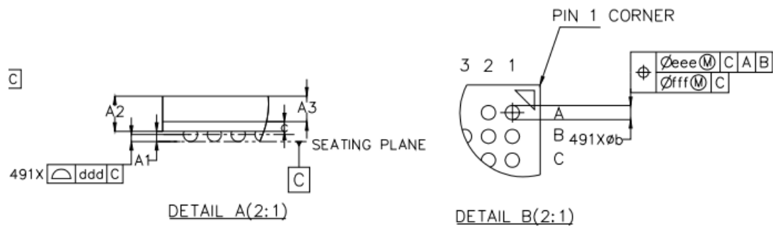
Fig. 2-3 RV1126B PKG Detail A&amp;B
