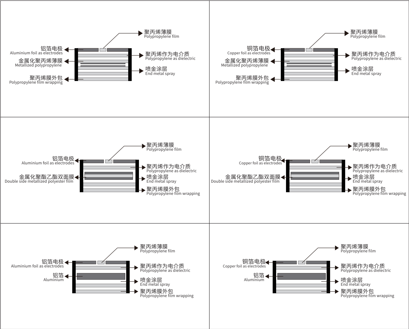
结构图.Construction Diagram
