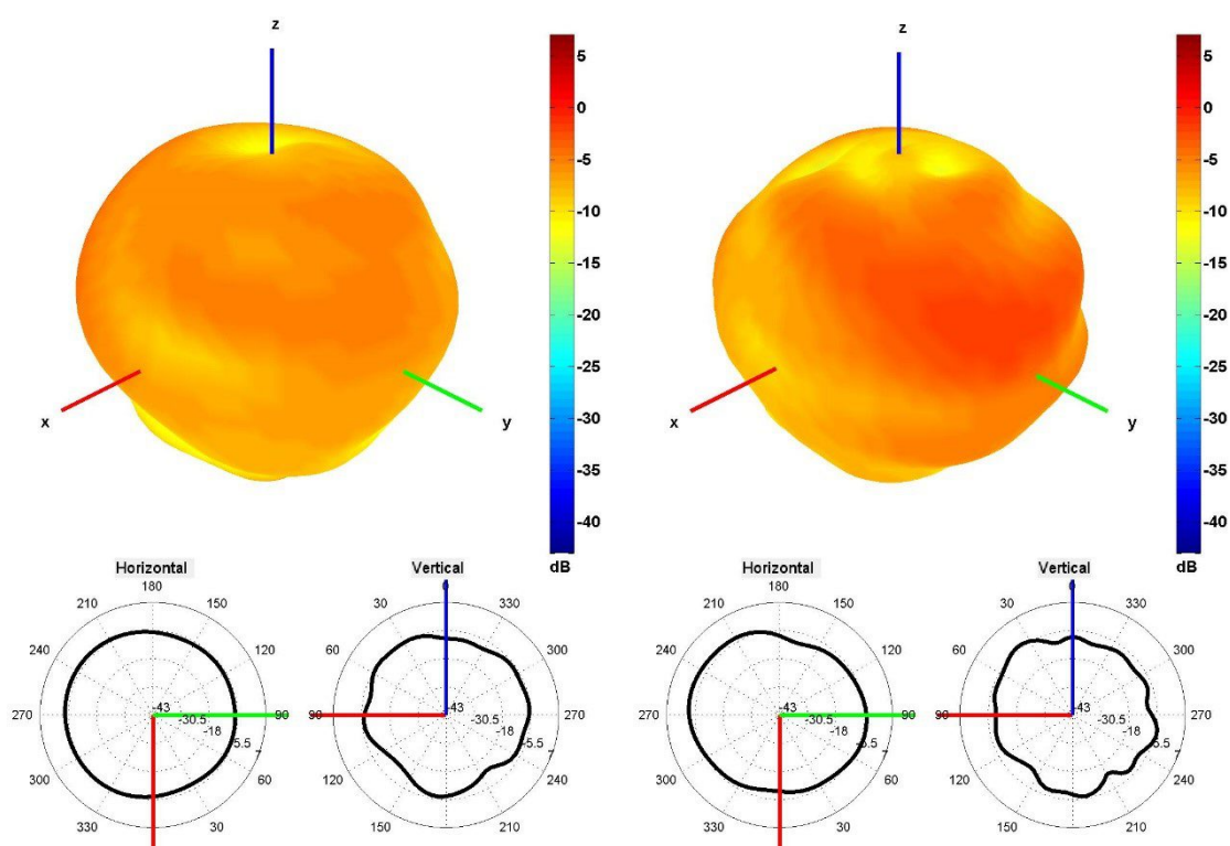
Cable 4: 5GNR
