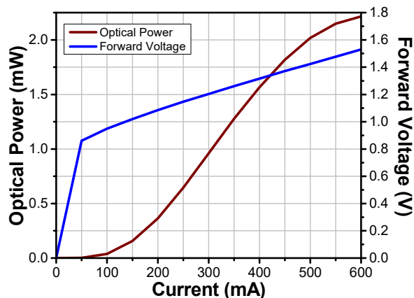
SLD1550P-A2 LIV
