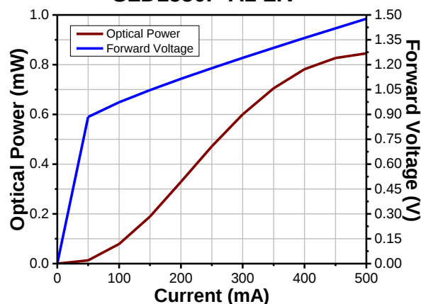
SLD1550P-A1 LIV
