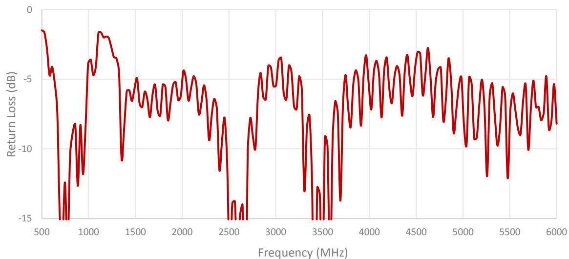
Cable 1: 5GNR
