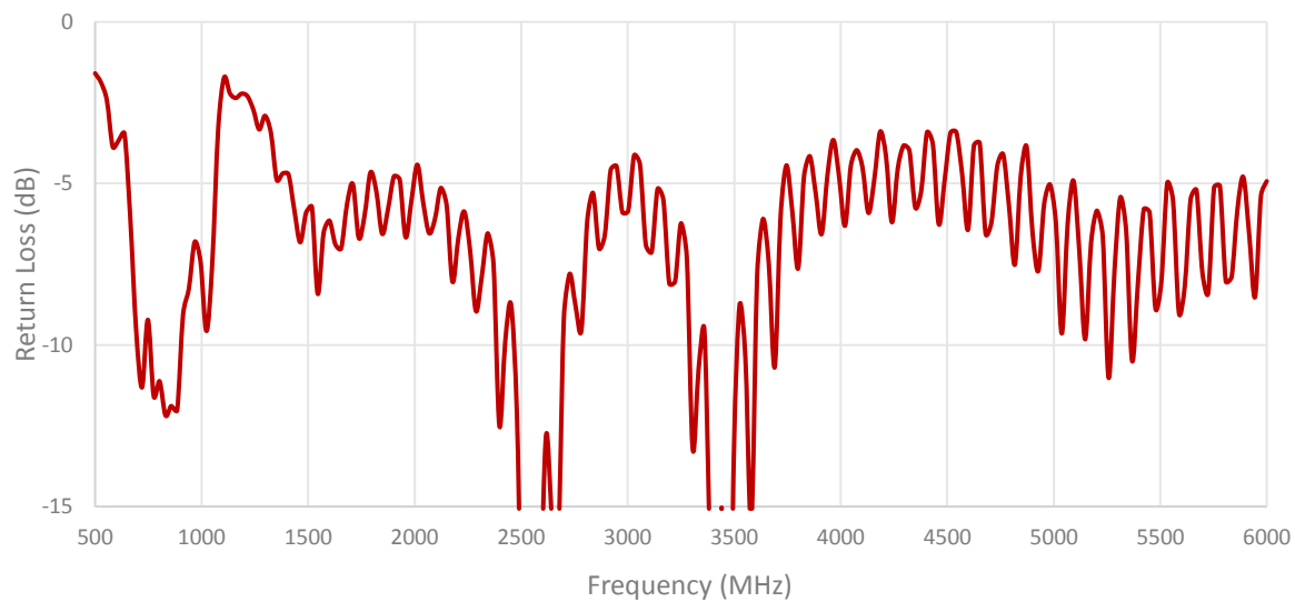
Cable 2: 5GNR
