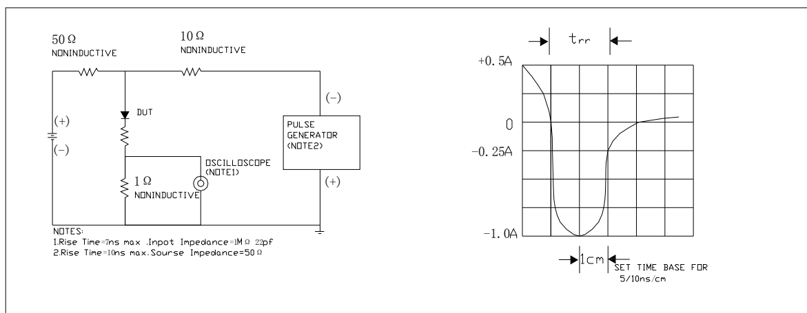
FIG.5 反向恢复时间试验电路及测试波形示意图
