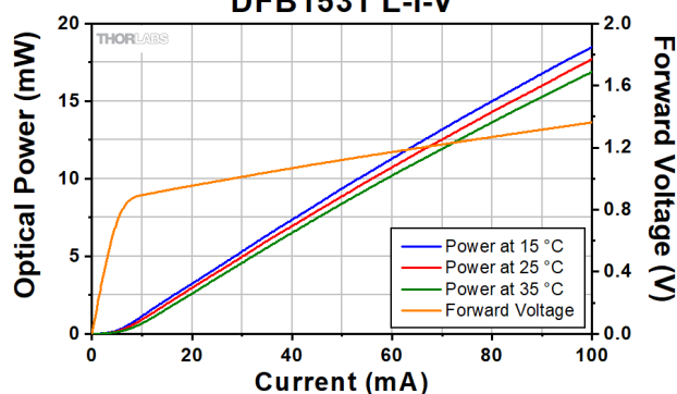
DFB1531 L-I-V
