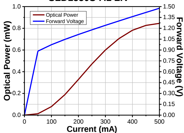
SLD1550S-A1 LIV
