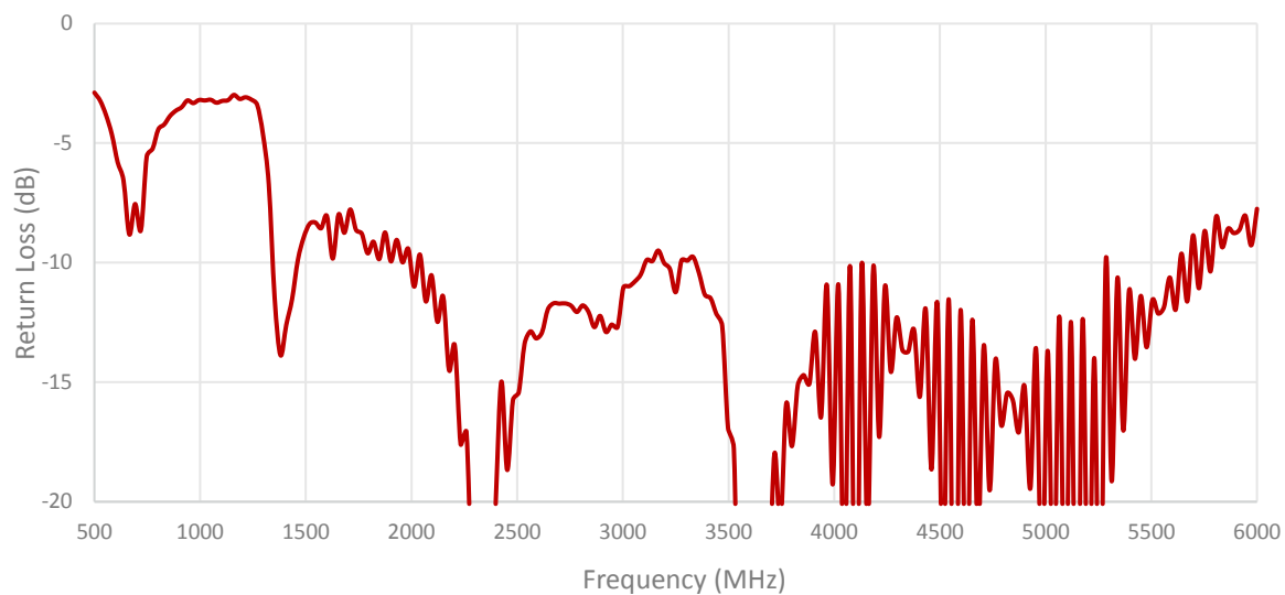
Cable 3: 5GNR
