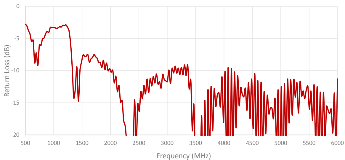
Cable 4: 5GNR
