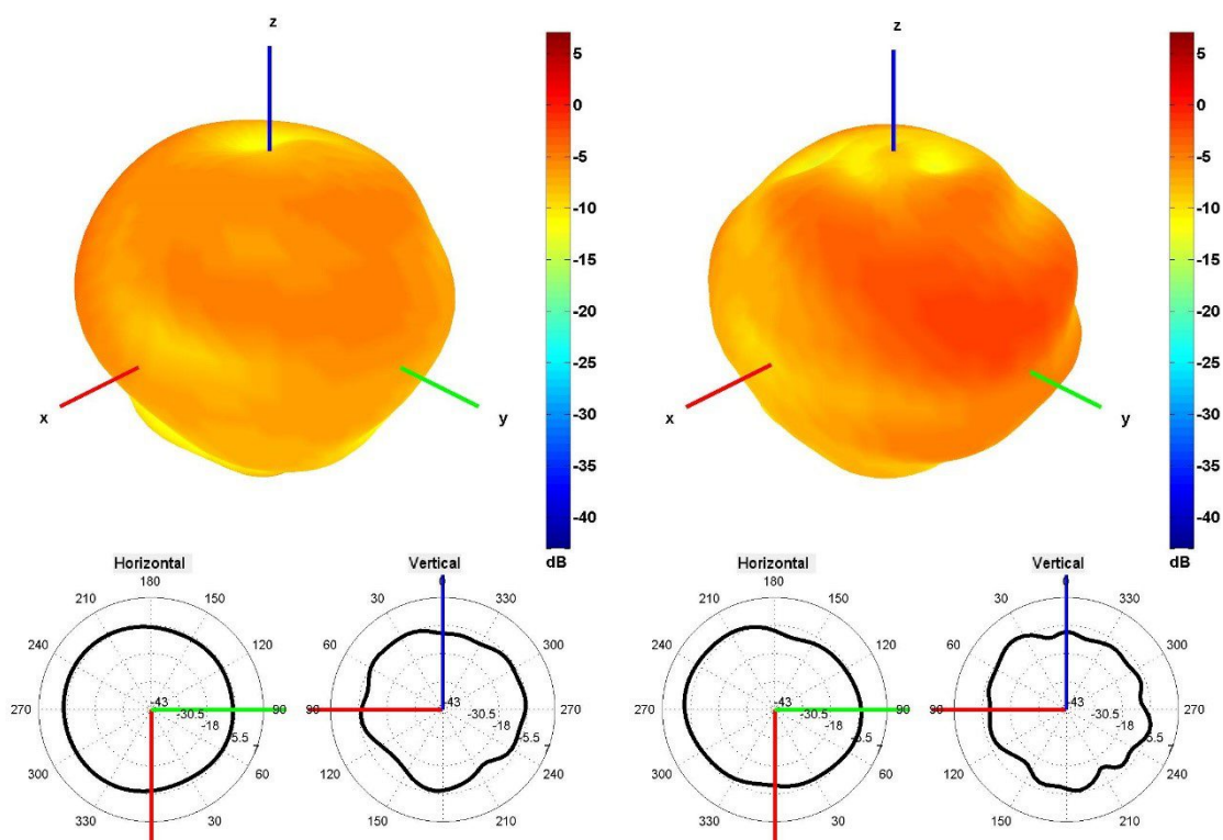
Cable 4: 5GNR
