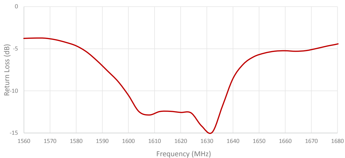
Cable 2: IRIDIUM
